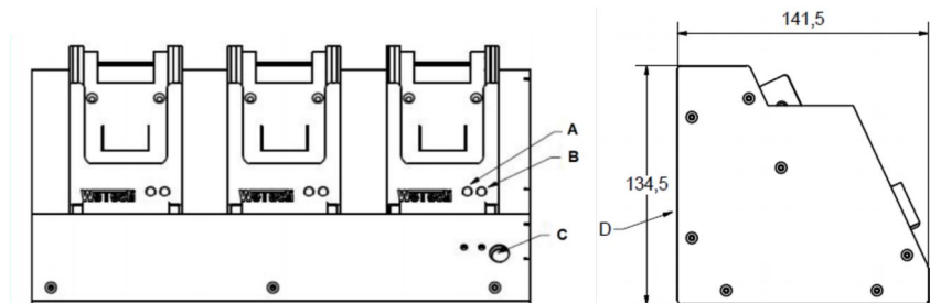
Schemazeichnung DC681-3-12V
